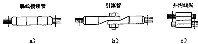
图 C.2 不受拉的接续金具的电位测点
