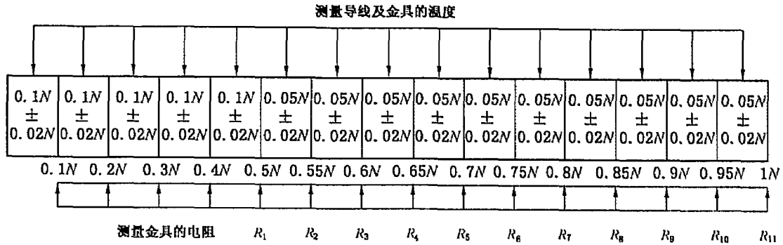
图 E.1 热循环试验程序明细表
