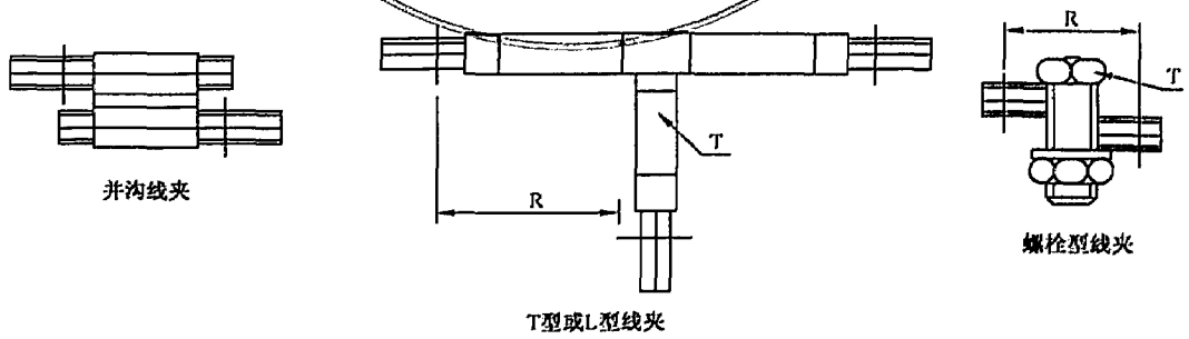
图 A.5 分支式接续管
