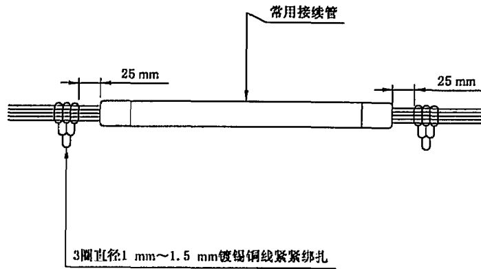
图 D.1 电位测点
